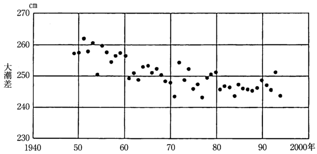
図16 伊勢湾名古屋港における大潮差（大潮の時の潮の満ち引きによる水位差の平均値）の経年変化 伊勢湾の埋立ての結果、年々潮汐が減少している。
